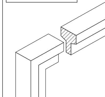
パネル枠 断面形状
