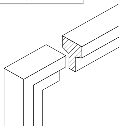
パネル枠 断面形状
