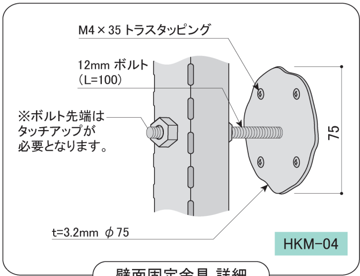
壁面固定金具 詳細
