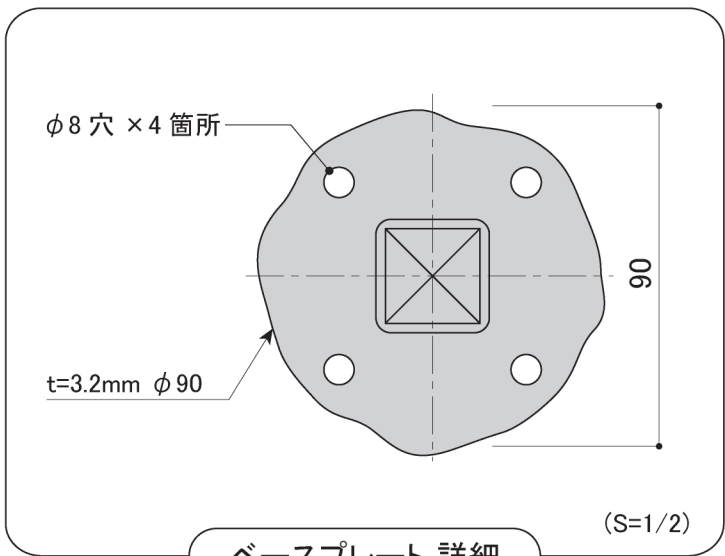
ベースプレート 詳細
