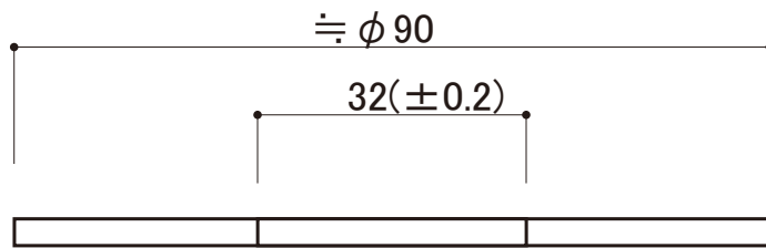
断面図 S=1/1
