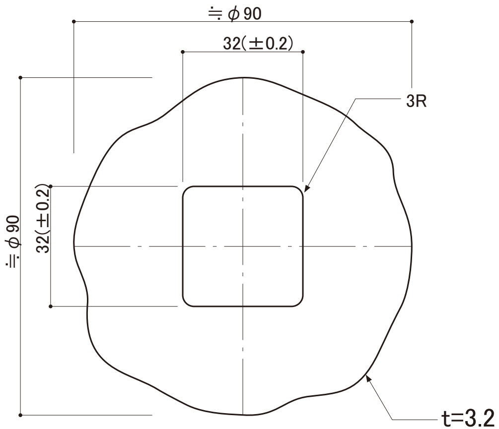
断面図 S=1/1
