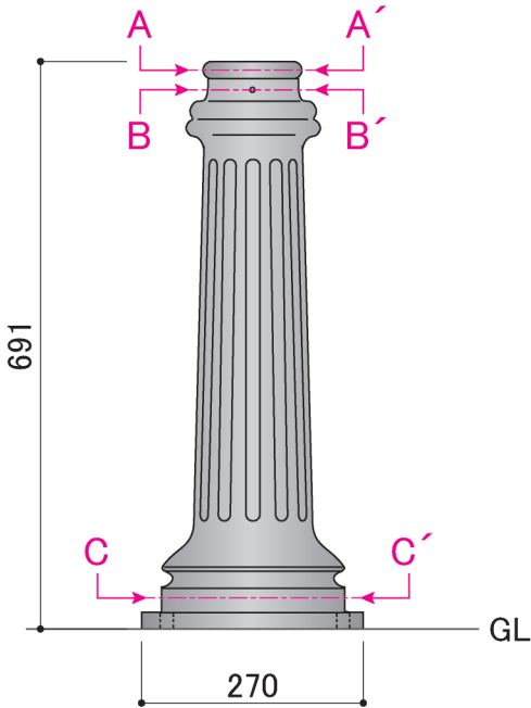
立面図 S=1/10
