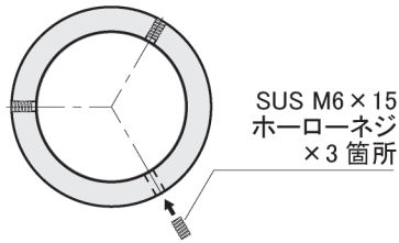
B-B' 断面図
