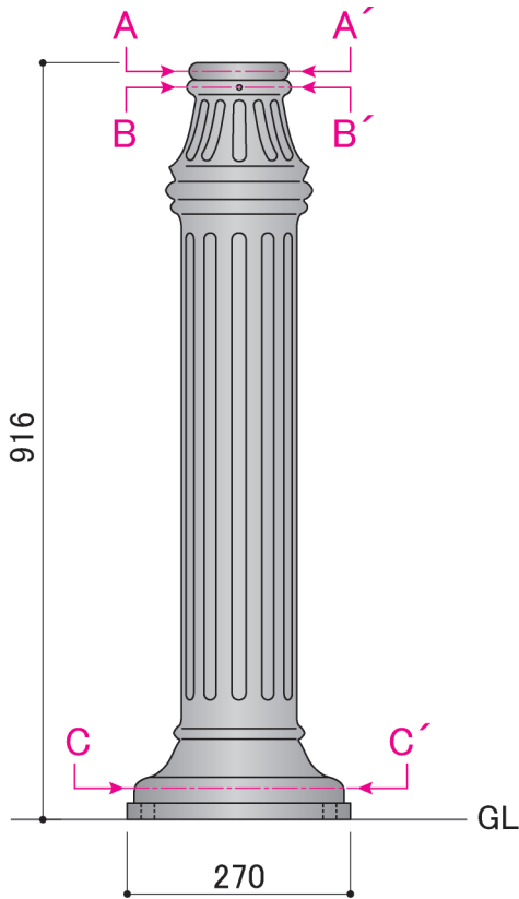
立面図 S=1/10
