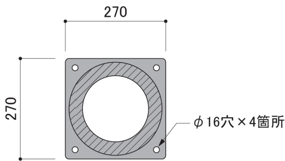
C-C' 断面図
