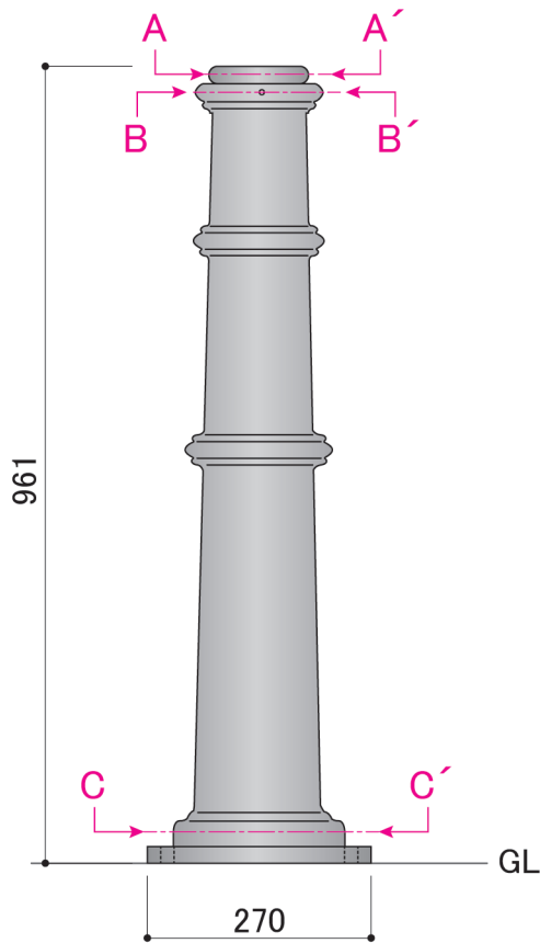
立面図 S=1/10
