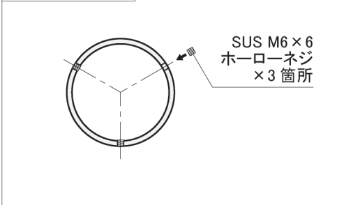
C-C' 断面図 <S=1/5>
