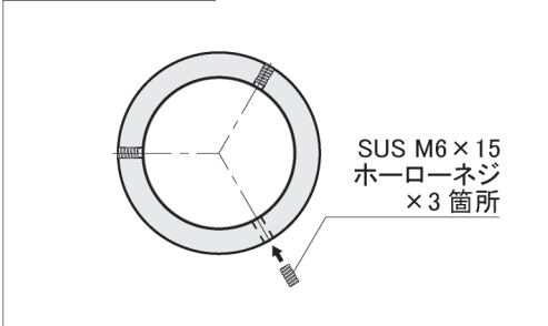
B-B' 断面図 <S=1/5>
