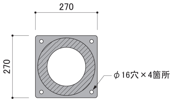
C-C' 断面図
