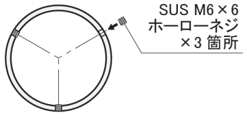
B-B' 断面図
