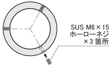
B-B' 断面図
