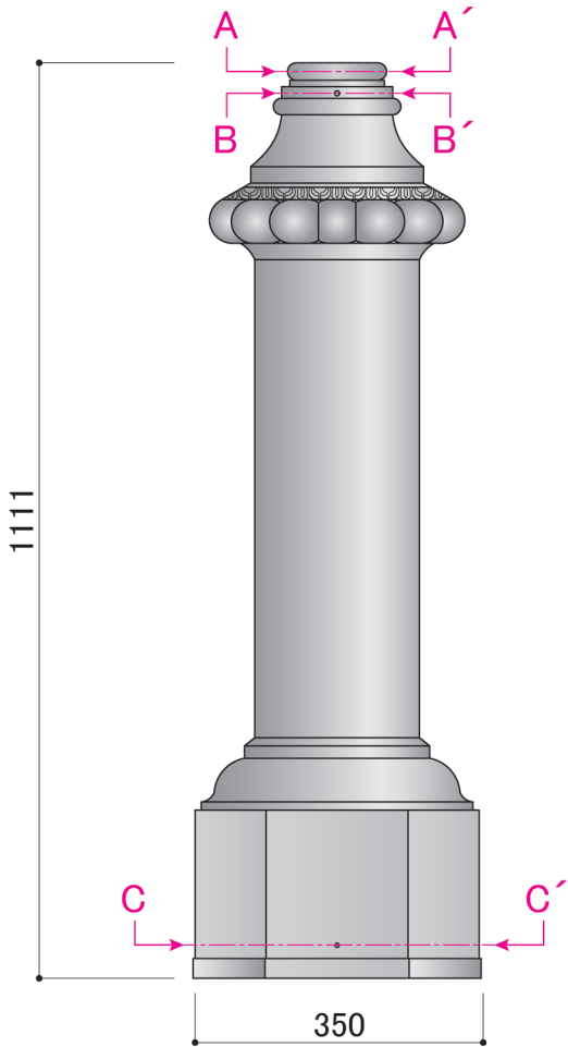
正面図
