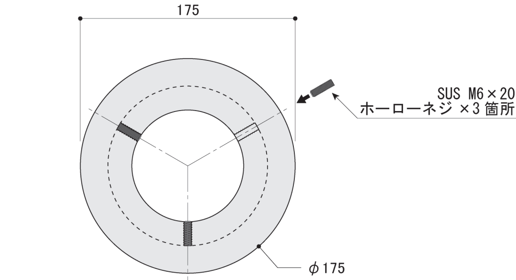
平面図
