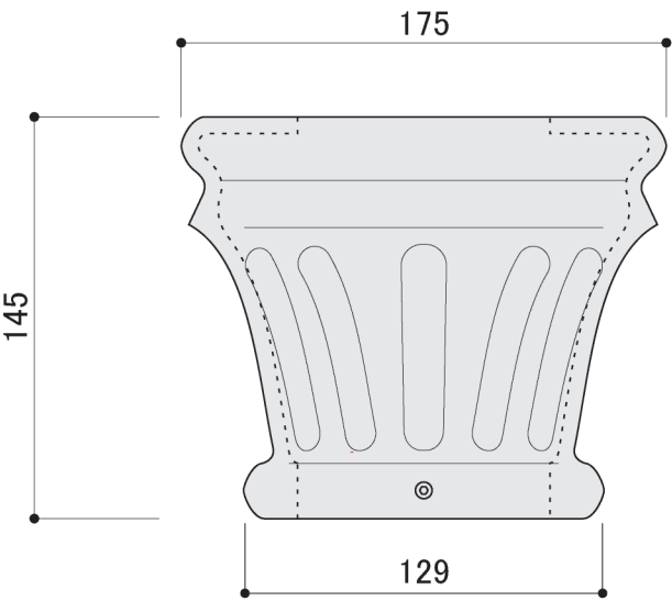
立面図
