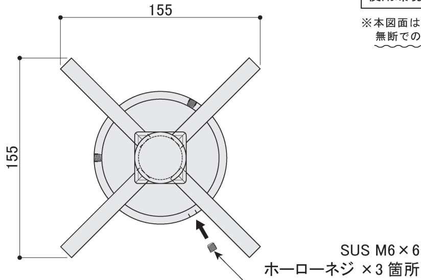
平面図 S=1/3
