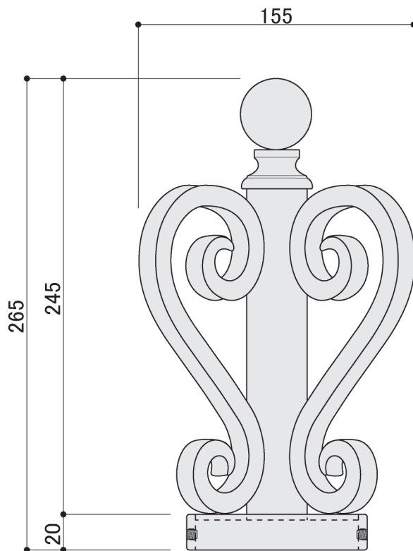
立面図 S=1/3
