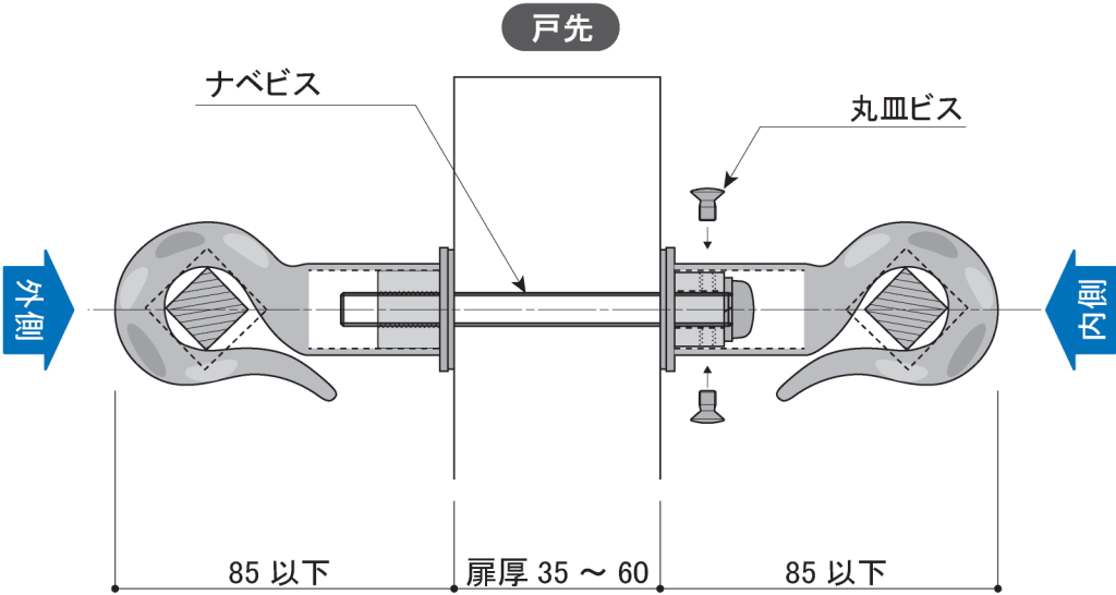
平断面詳細図 S=1/2
