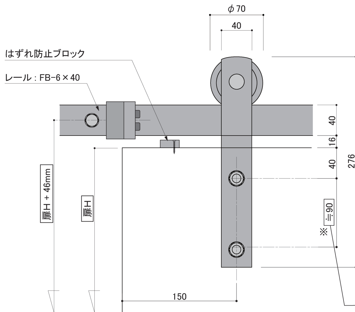
全体姿図 S=1/20
