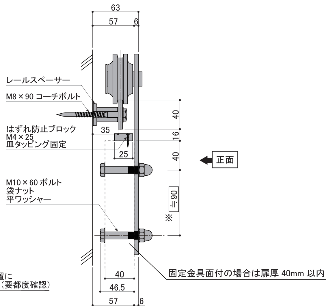
側面図 S=1/3
