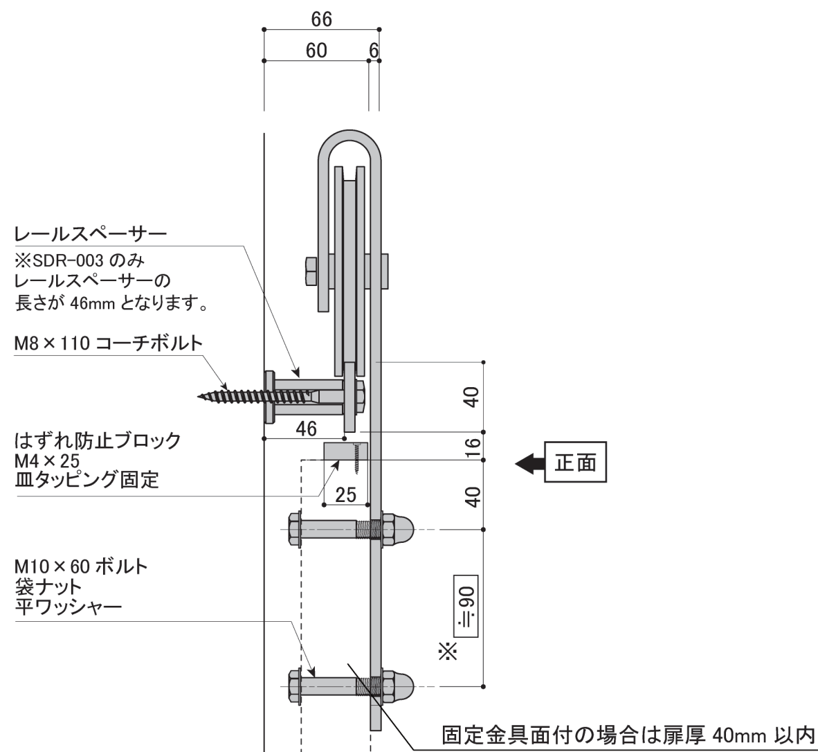
側面図 S=1/3
