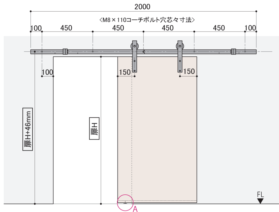
全体姿図 S=1/20
