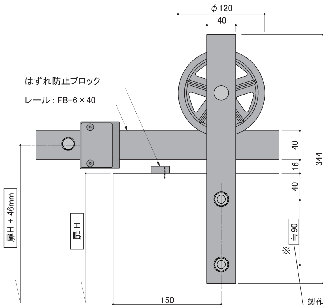
正面図 S=1/3
