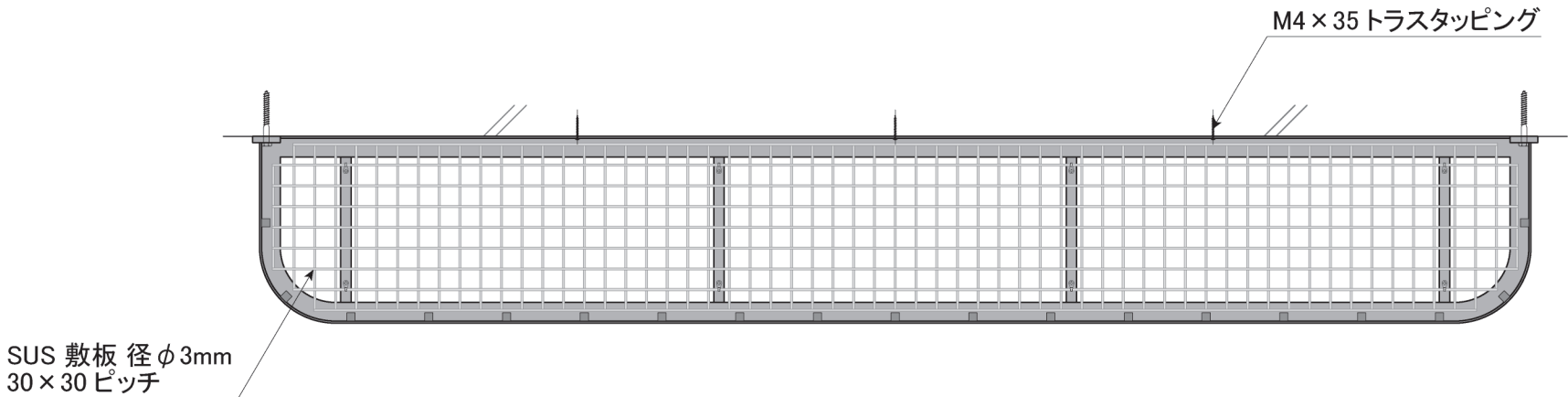
B 平断面 底面部
