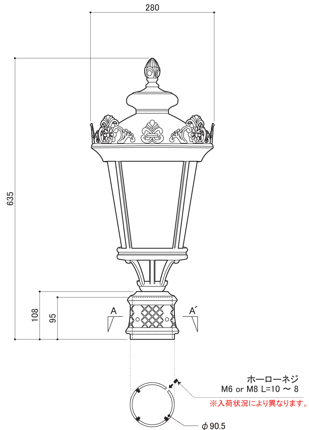
A-A' 平断面図
