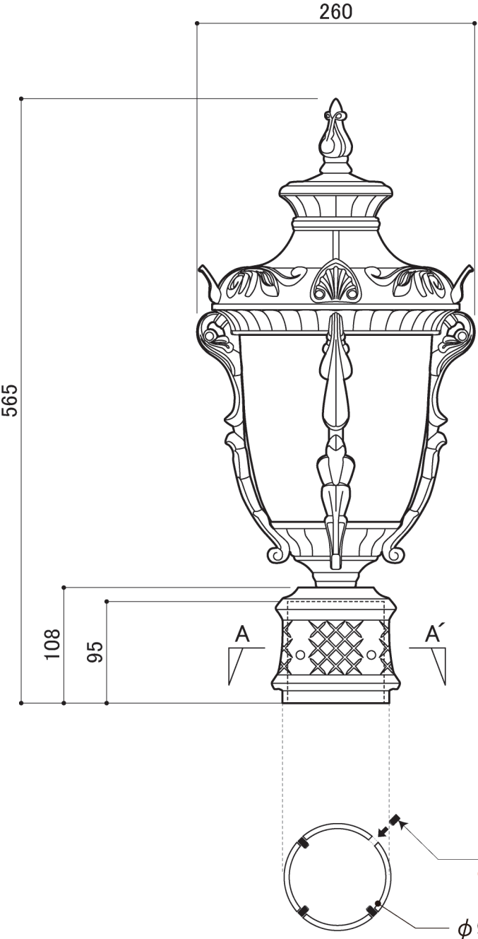
A-A' 平断面図
