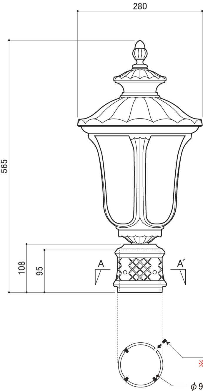
A-A' 平断面図
