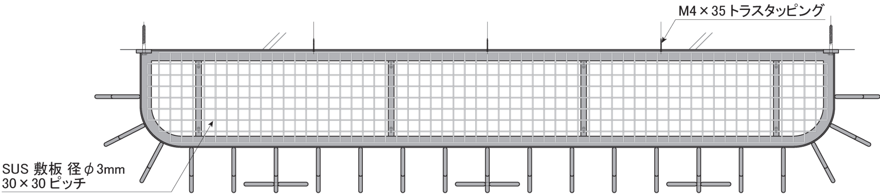
B 平断面 底面部
