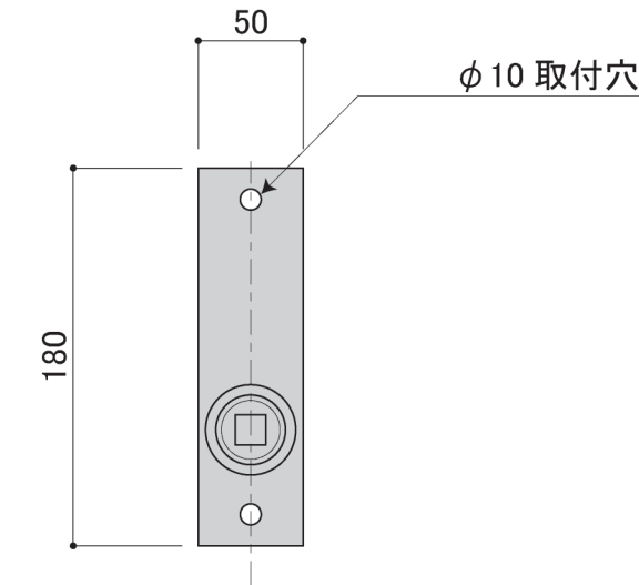
A-A' 方向側断面図 S=1/4
