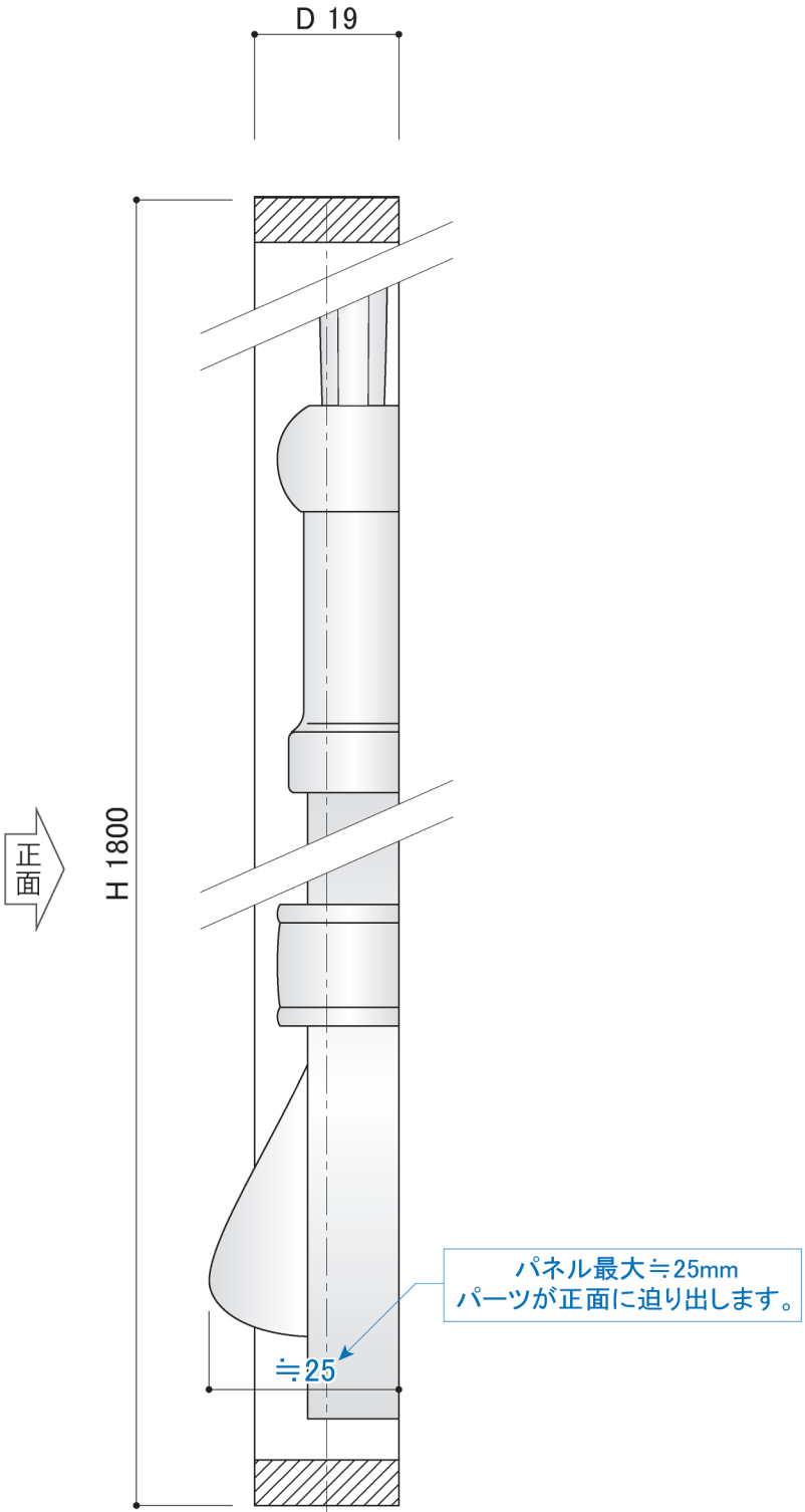
〈側断面詳細図 S=1/1〉
