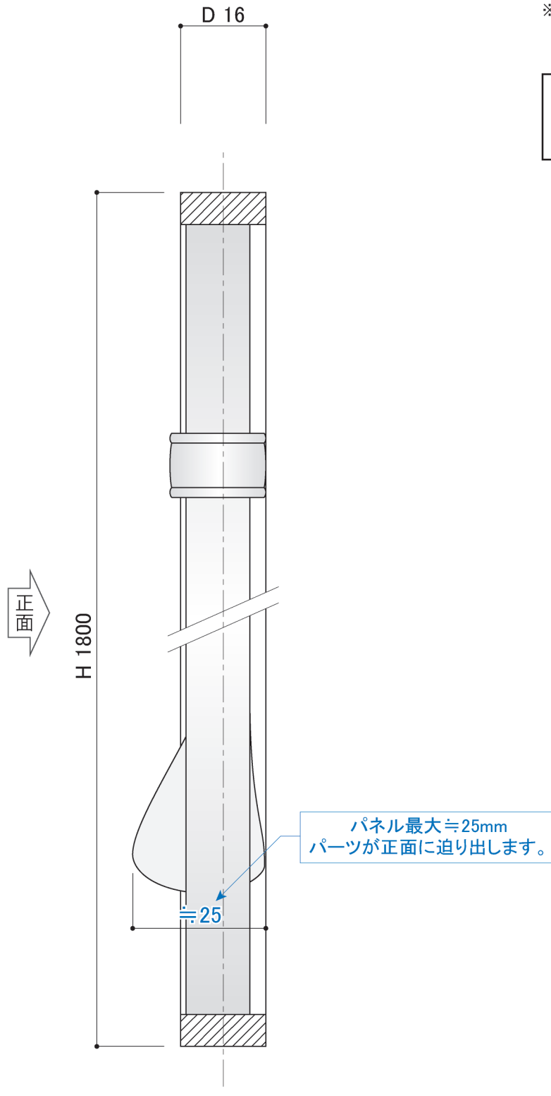
〈側断面詳細図 S=1/1〉
