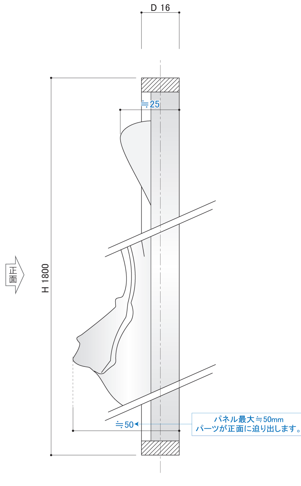
〈側断面詳細図 S=1/1〉
