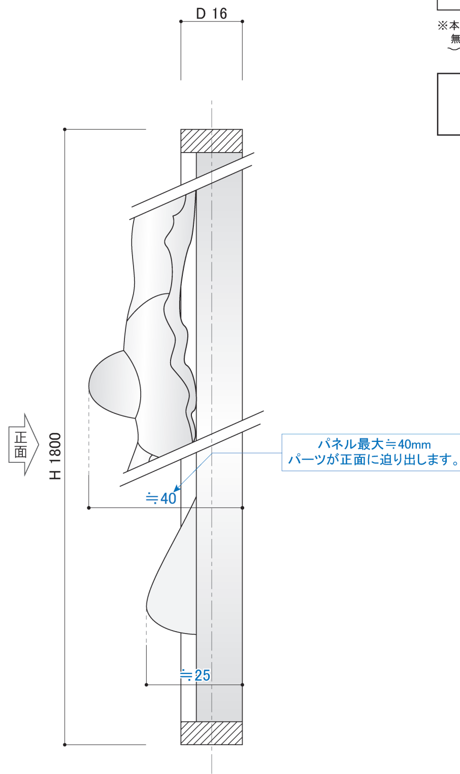
〈側断面詳細図 S=1/1〉
