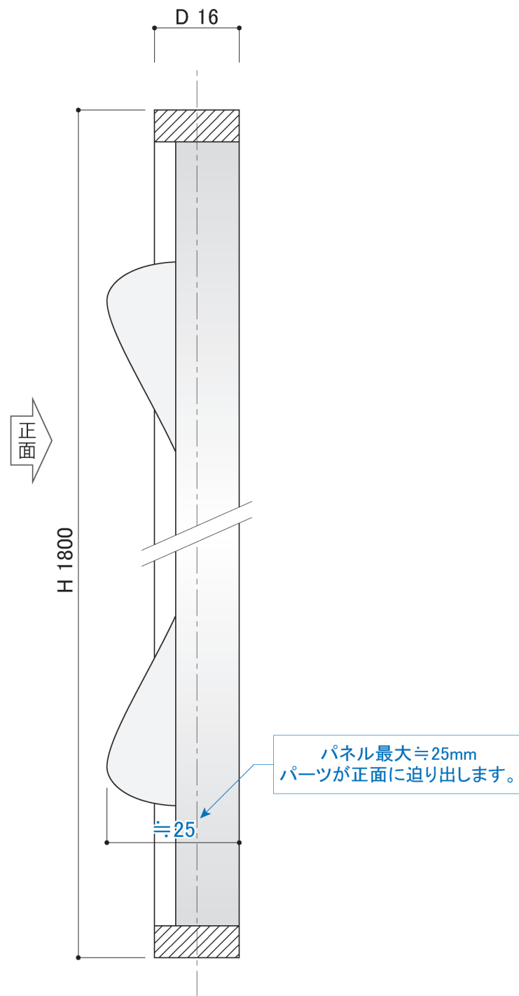
〈側断面詳細図 S=1/1〉
