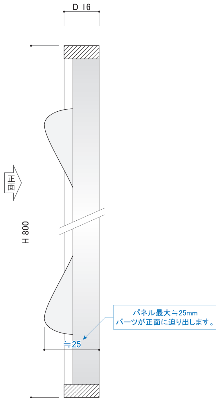
〈側断面詳細図 S=1/1〉
