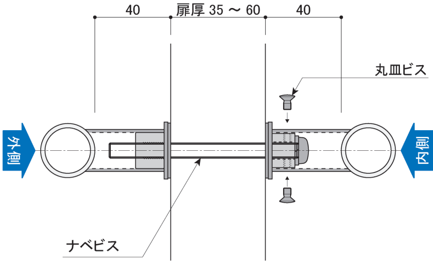
平断面詳細図 S=1/2
