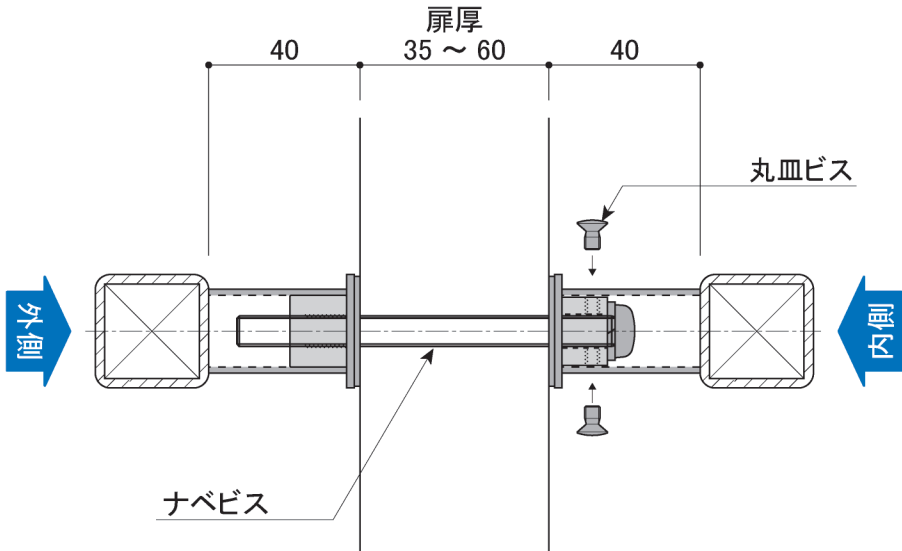
平断面詳細図 S=1/2
