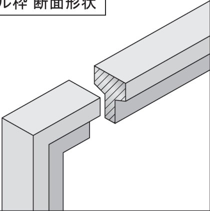
パネル枠 断面形状
