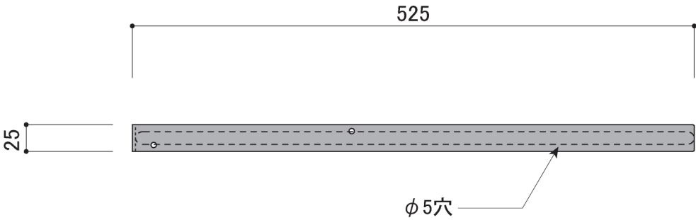
平面図 S=1/5
