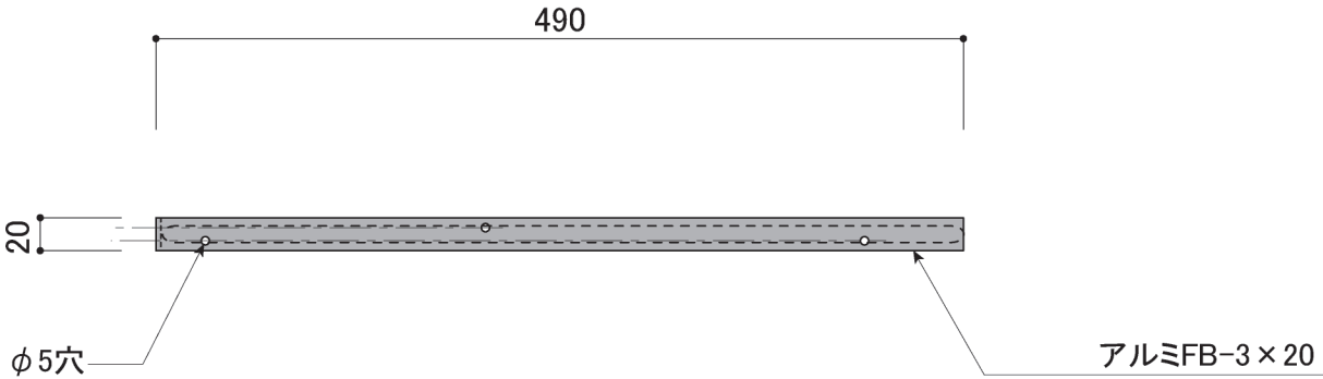
平面図 S=1/5
