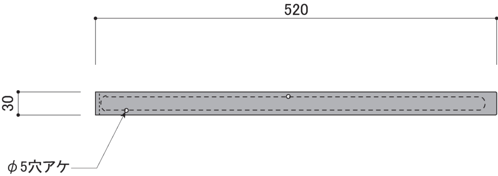
平面図 S=1/5
