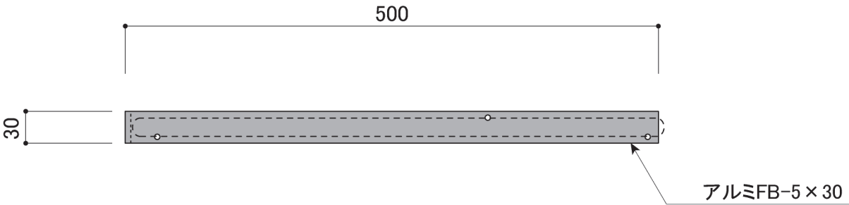
平面図 S=1/5
