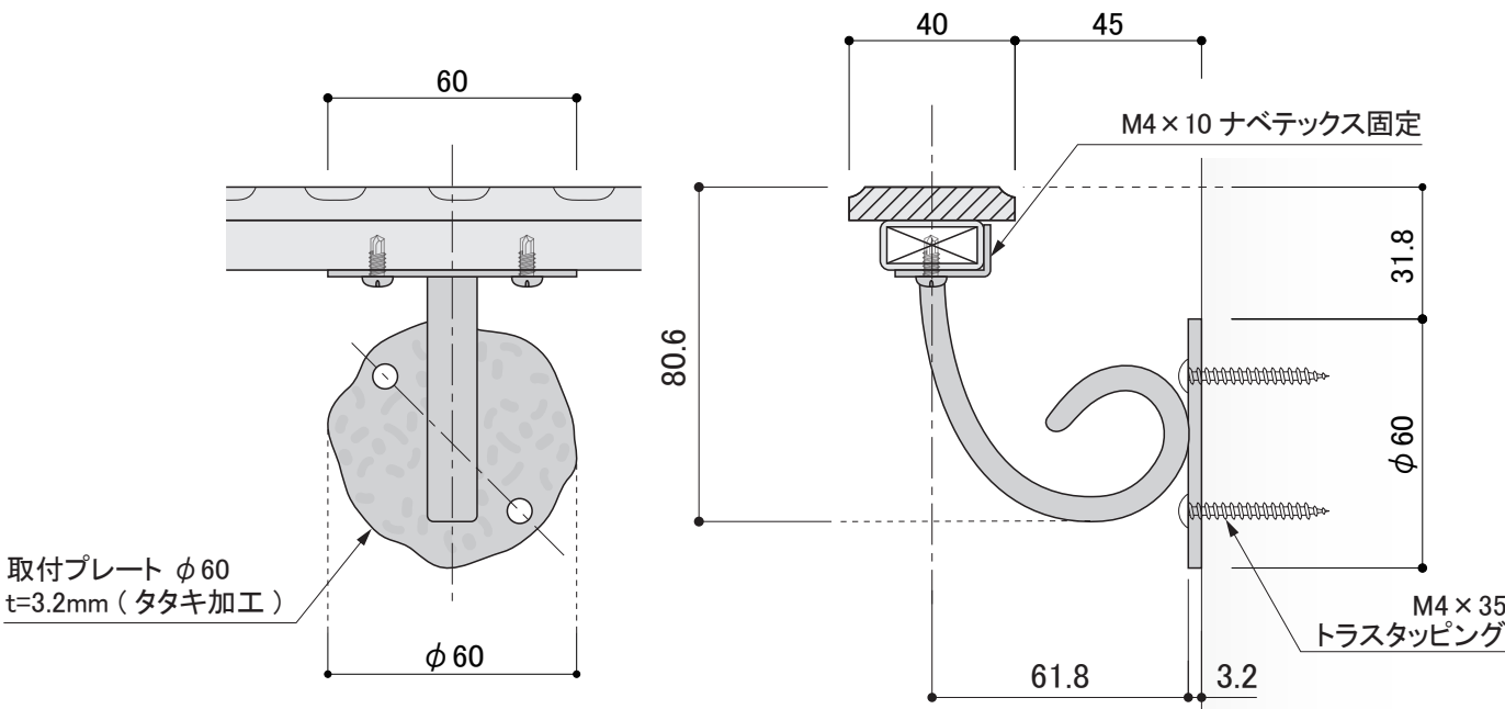
b : ブラケット詳細図 S=1/2
