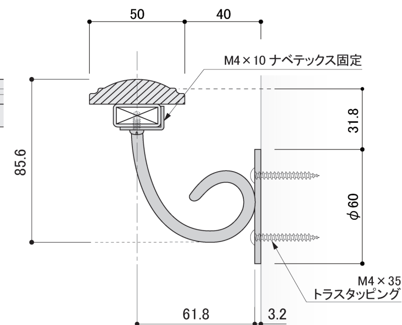
b: ブラケット詳細図 S=1/2
