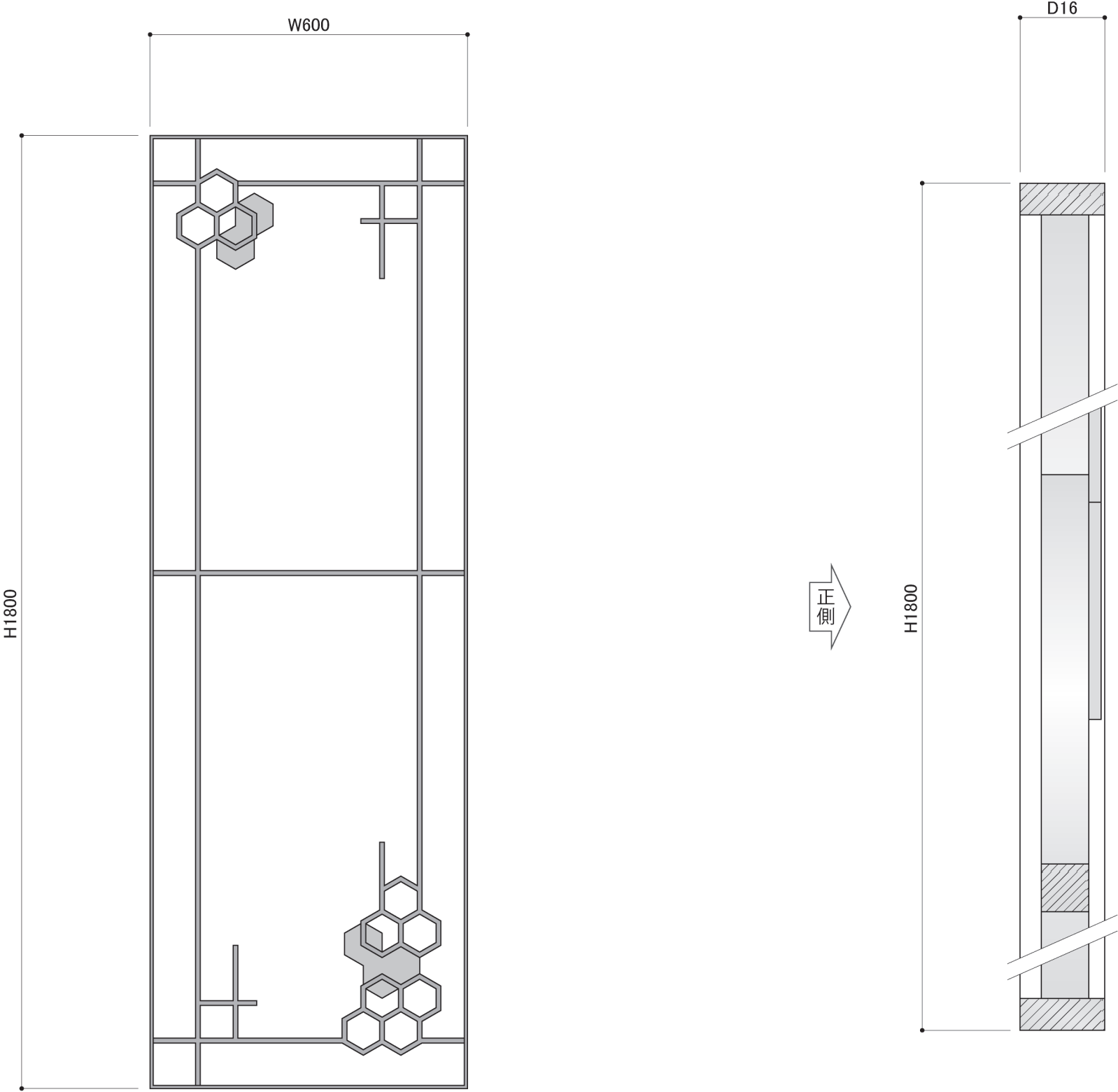
〈側断側詳細図 S=1/1〉
