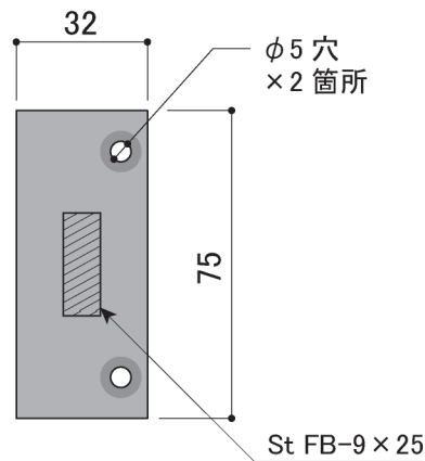
＜ベースプレート詳細 S=1/2＞
