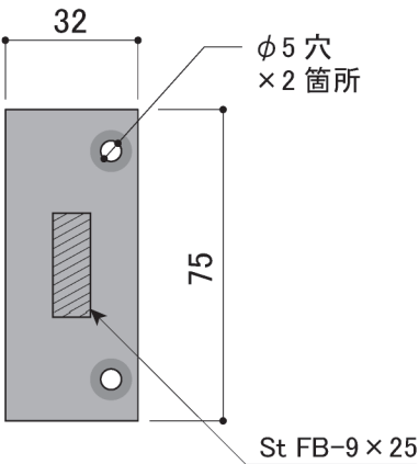
＜ベースプレート詳細 S=1/2＞
