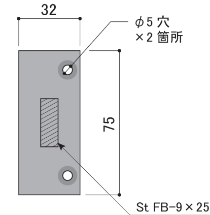
＜ベースプレート詳細 S=1/2＞
